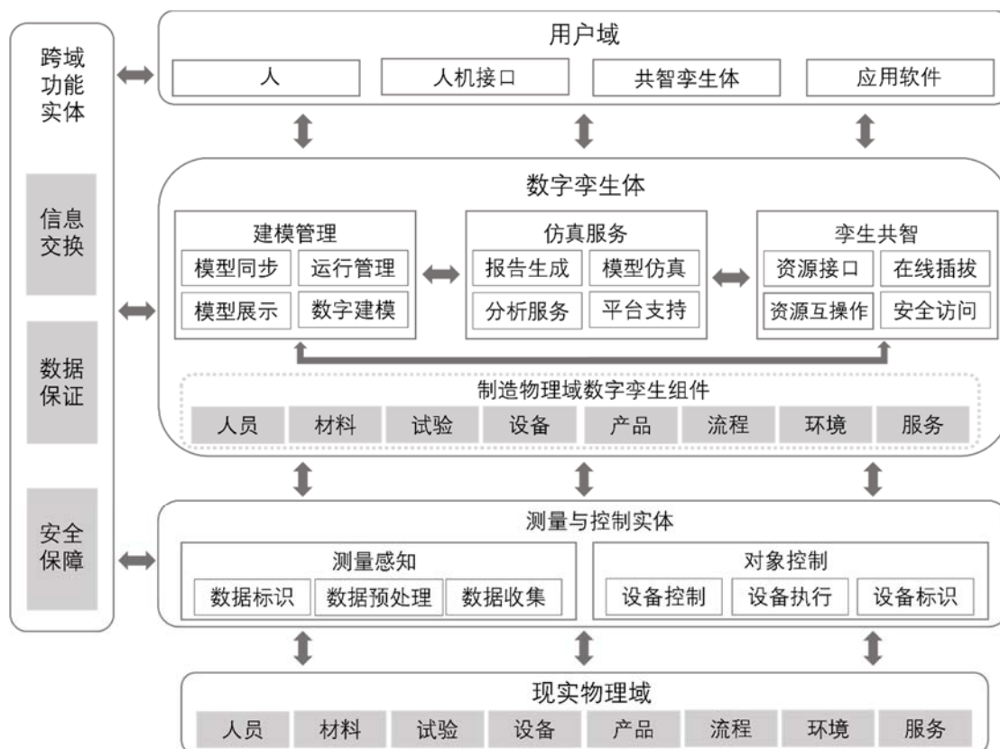
图 3-1 数字孪生制造参考技术架构
