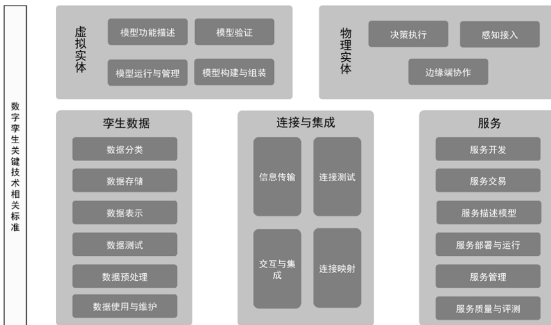
图 1-5 数字孪生关键技术相关标准
