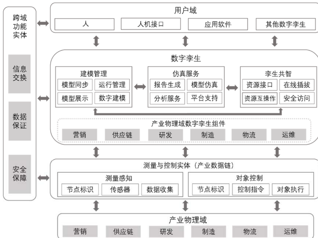
图 1-2 数字孪生系统通用参考架构
